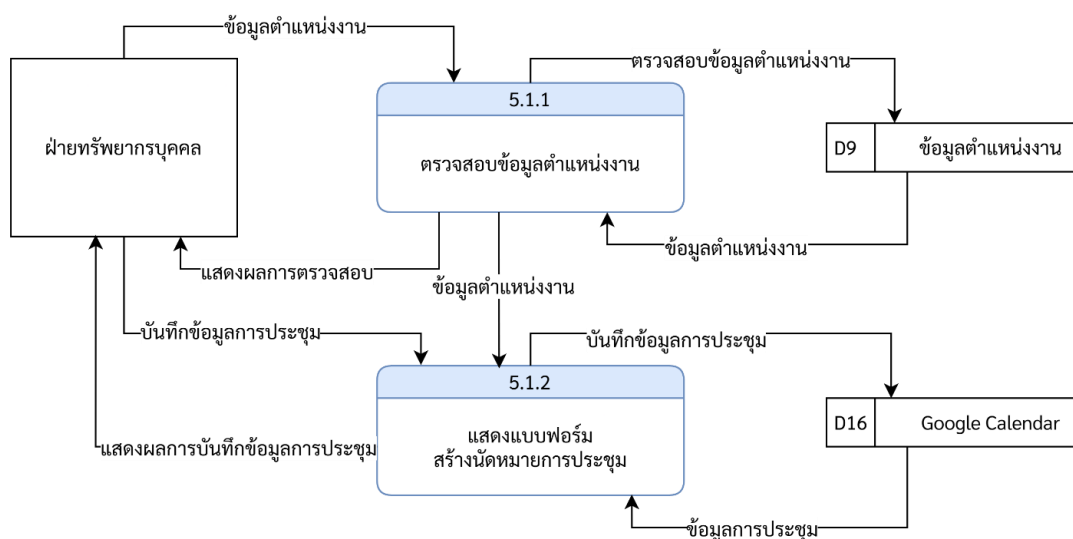
ภาพที่ 3-34 Data Flow Diagram Level 2 ของ Process การสร้างนัดหมายการประชุม (ฝ่ายทรัพยากรบุคคล)
