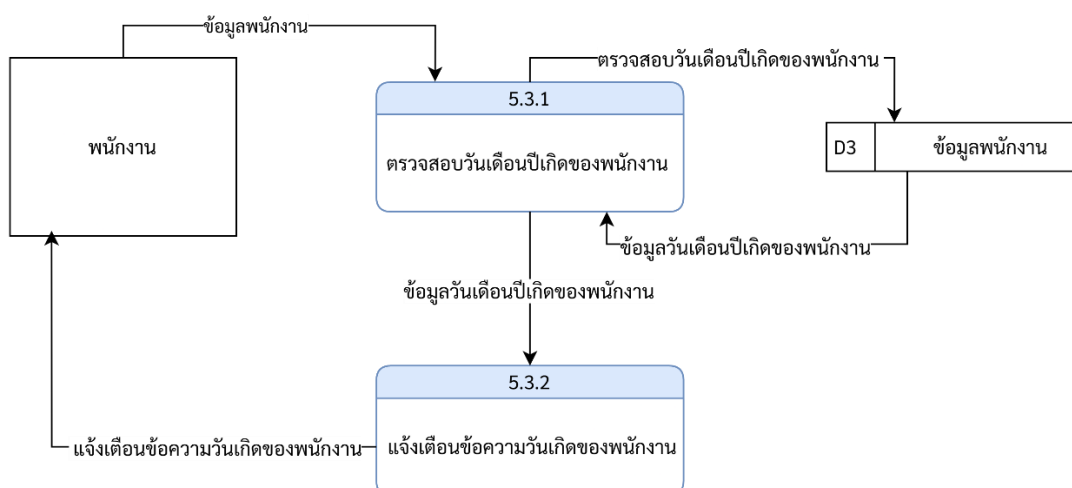
ภาพที่ 3-36 Data Flow Diagram Level 2 ของ Process การแจ้งเตือนวาระสำคัญ (เช่น วันเกิด) (พนักงาน)
