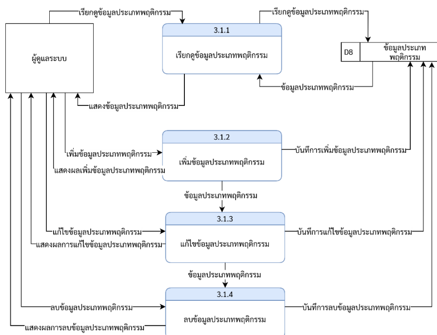
ภาพที่ 3-19 Data Flow Diagram Level 2 ของ Process การกำหนดประเภทและเกณฑ์การประเมินพฤติกรรม (ผู้ดูแลระบบ)
