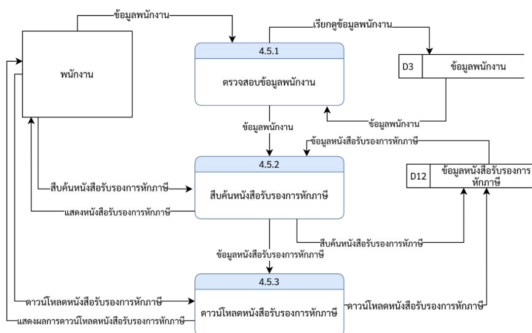
ภาพที่ 3-30 Data Flow Diagram Level 2 ของ Process การดาวน์โหลดหนังสือรับรองการหักภาษี (พนักงาน)
