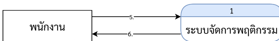
ภาพที่ 3-18 Data Flow Diagram ระบบจัดการพฤติกรรม Level 1 (พนักงาน)
